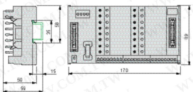
ABE 7TES160
